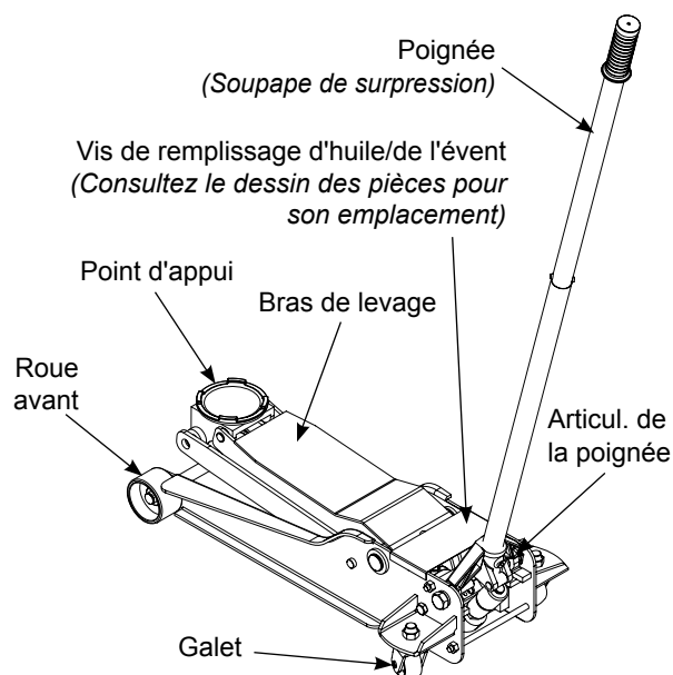
Figure 1 : Pièces d'un cric typique
