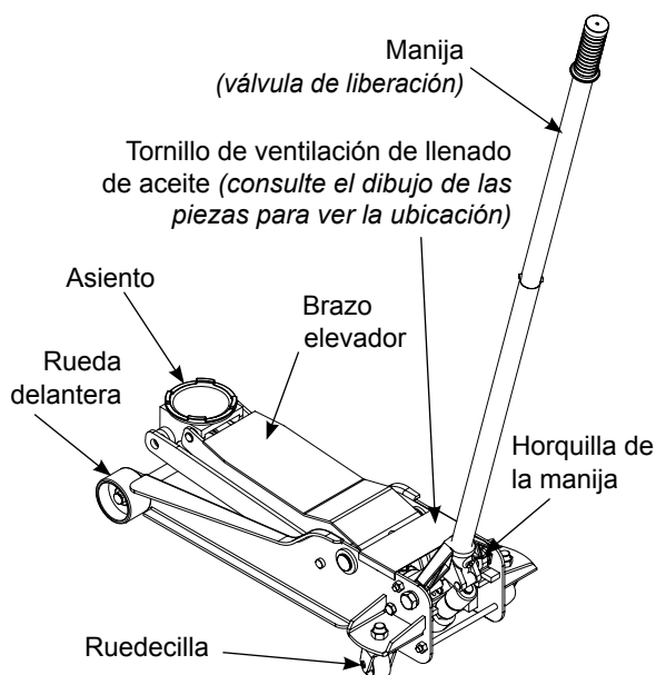
Figura 1: Nomenclatura habitual de un gato
