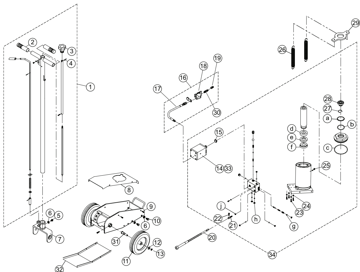
Figure 3 : Illustration des pièces de rechange du modèle 23301C
